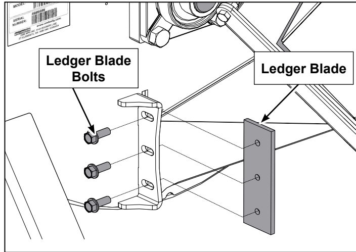
Fig. 27 LEDGER BLADE
