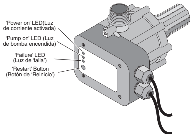
Figura 4 – Tablero de control de controlador automático de presión
