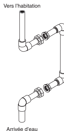
Figure 3 : Branchement type de la tuyauterie de dérivation pour permettre la dépose de la pompe au cas où elle devrait être réparée, sans avoir à fermer toute l'alimentation d'eau de l'habitation.
