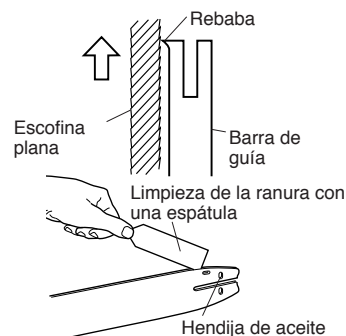
Figura 22 - Mantenimiento de la barra de guía
