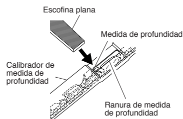
Figura 25 - Calibrador de medida de profundidad en la cadena
