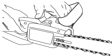
Figura 9 - Presione la Ampolla de Apriete en la Tapa del Aceite para Aceitar la Cadena
