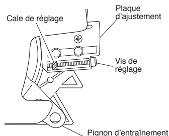
Figure 5 - Emplacement des pièces pour l'assemblage du guide-chaîne
