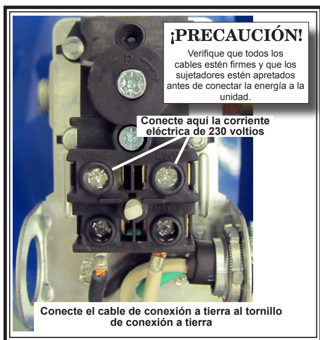
Fig. 1 Conexiones eléctricas para el modelo 1312101159
