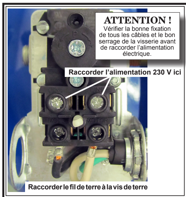
Fig. 1 Raccordements électriques du modèle 1312101159
