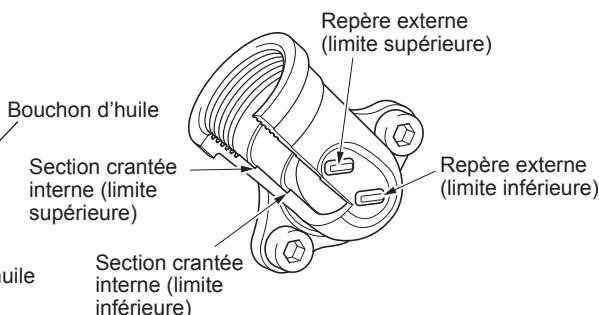
Fig. 2 Tuyau d'huile
