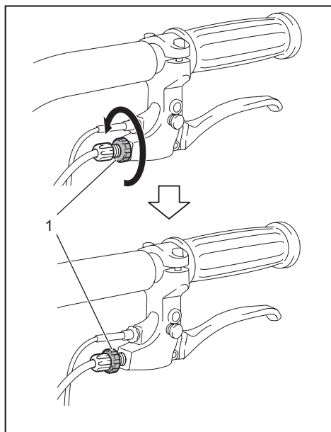
► 1. Fixing nut
