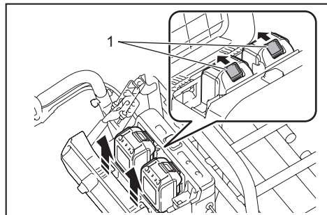
► 1. Botón
