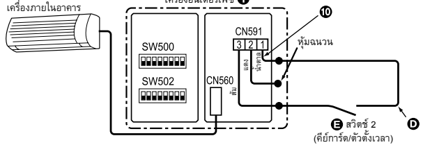
การเชื่อมต่อรีโมทคอนโทรลและตัวตั้งเวลา
