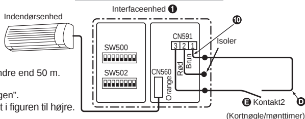
Forbindelse af kortnøgle og mønttimer
