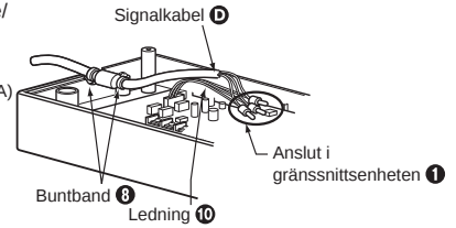
Kortnyckel timer-anslutning
