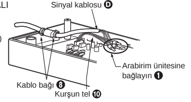
Kart anahtar bobin zamanlayıcı bağlantısı
