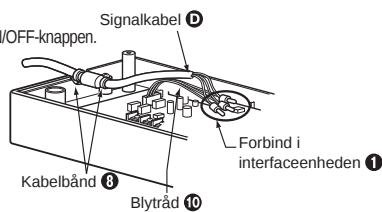
Forbindelse af kortnøgle og mønttimer
