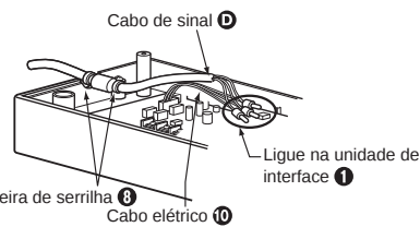
Ligação da chave de cartão ou temporizador de moeda
