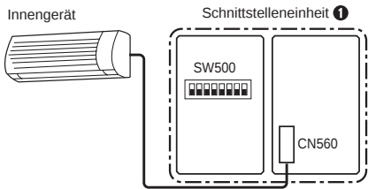
Konfiguration bei der Verwendung des Ein-/Ausschaltens mit Spannung
