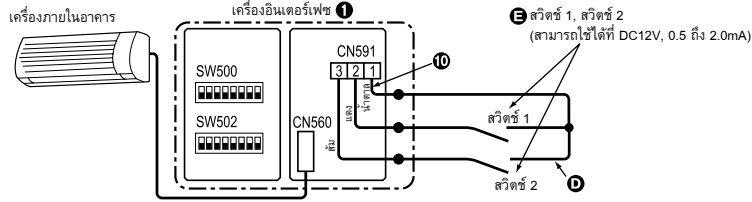
การเชื่อมต่อรีโมทคอนโทรลและตัวตั้งเวลา
