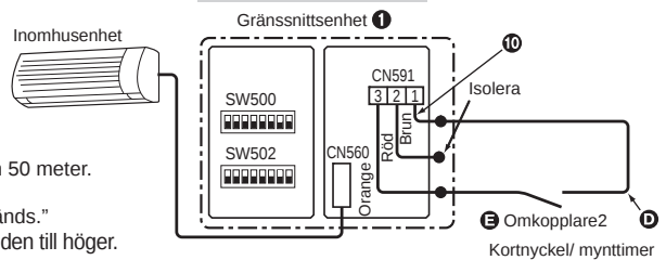
Kortnyckel timer-anslutning
