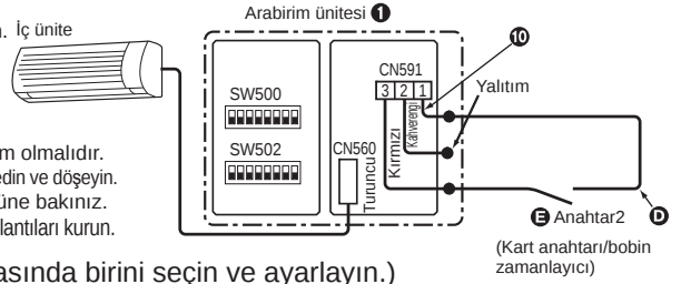
Kart anahtar bobin zamanlayıcı bağlantısı
