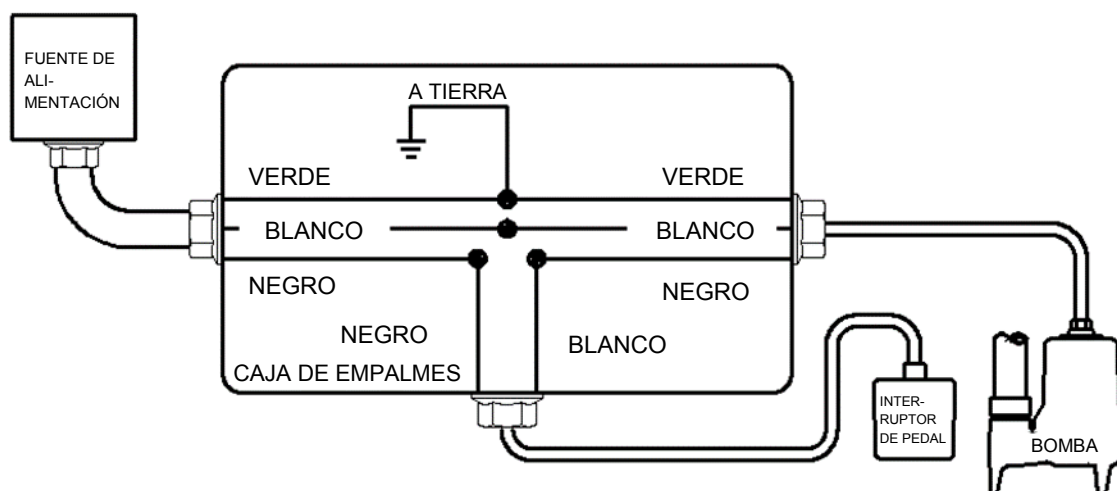
Fig. 6 – Cableado directo de bomba(s) automática(s) monofásicas de 120 V o 208-230 V
