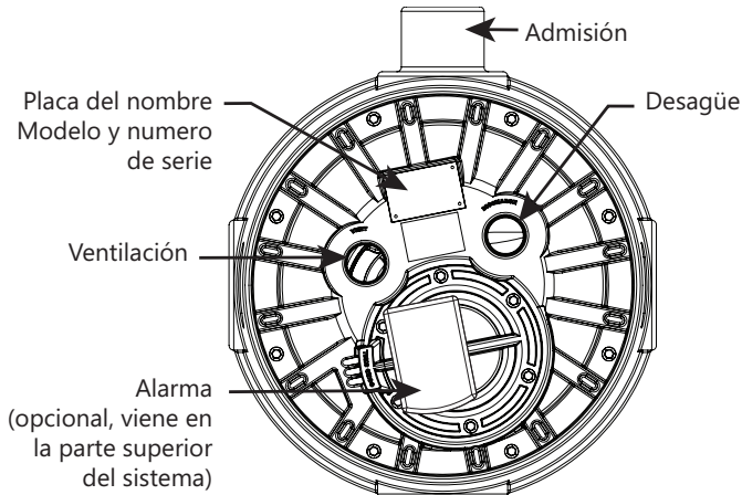
Figura 5. Cubierta serie 370
