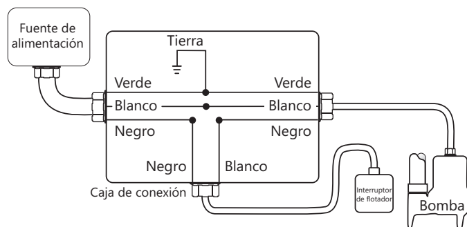
Figura 12. Cableado directo de 115V o 208V/230V, 1PH, bombas automáticas
