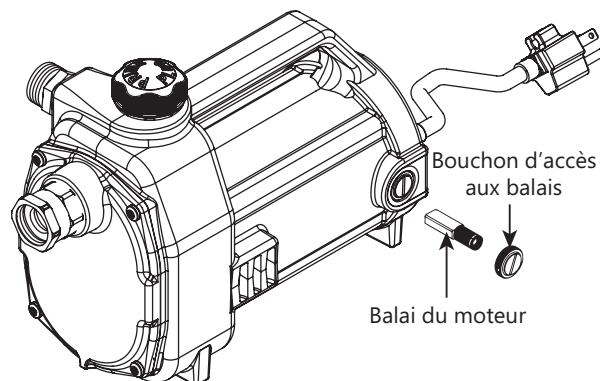
Figure 3. Brosse du moteur (un seul côté montré)
