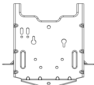
BARRE D'ATTELAGE B (INCLINÉ)
