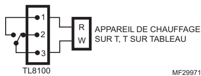
Fig. 10. Schéma de câblage pour un appareil de chauffage de 24 V c.a. ou un tableau de zonage à eau chaude.
