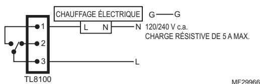
Fig. 4. Schéma de câblage pour un chauffage électrique sur tension secteur.
