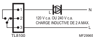
Fig. 3. Schéma de câblage pour un circulateur sur tension secteur.
