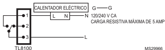
Fig. 4. Diagrama de cableado de un calentador eléctrico de voltaje de línea.
