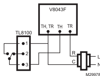
Fig. 8. Schéma de câblage d'une vanne de 24 V c.a. V8043F.
