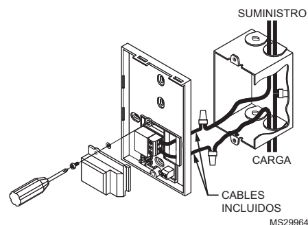
Fig. 2. Trazado de los cables hacia el termostato.
