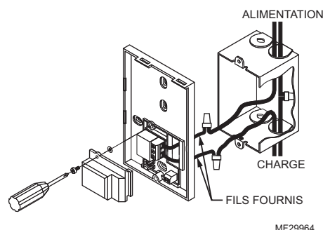
Fig. 2. Acheminement des fils vers le thermostat.
