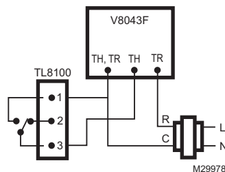
Fig. 8. Diagrama de cableado de la V8043F de 24 V CA.
