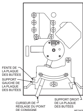
Fig. 2. Thermostat sans son couvercle.
