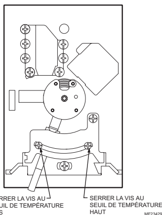
Fig. 3. Positionnement des butées de réglage sur le thermostat.
