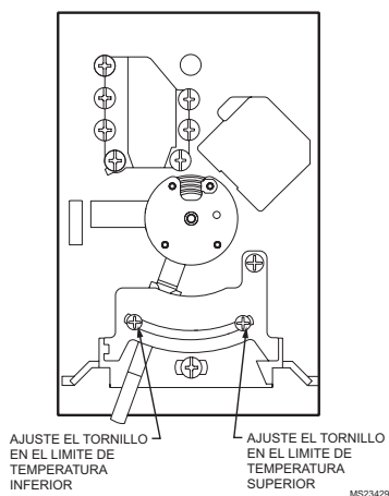
Fig. 3. Alineación del tope para rangos con el termostato.
