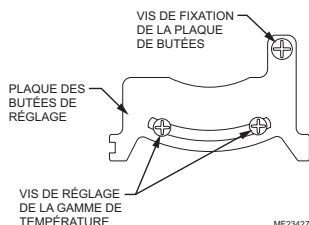
Fig. 1. Plaque de butées de réglage et vis.
