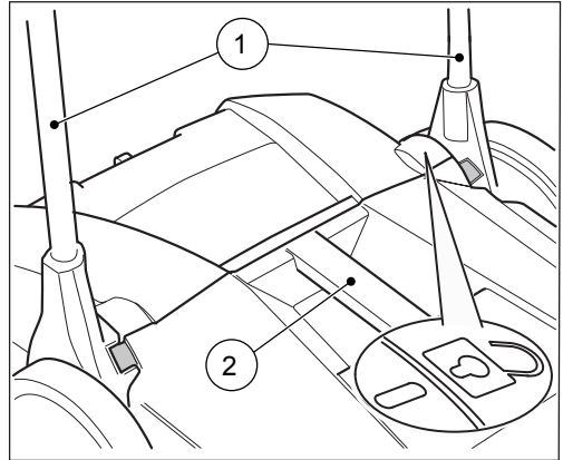
Abb. 11: Freigabeposition Kehrgutbehälter
