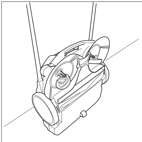
Abb. 5: Aufbewahrungposition
