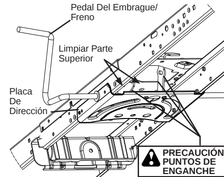
SISTEMA DE DIRECCIÓN, SALPICADERO, GUARDABARROS Y SEGADORA NO MOSTRADOS
