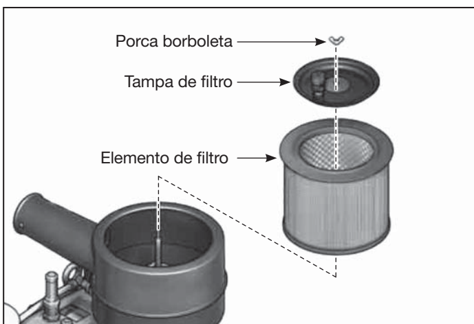
Figura 14 - Filtro de admissão de ar
