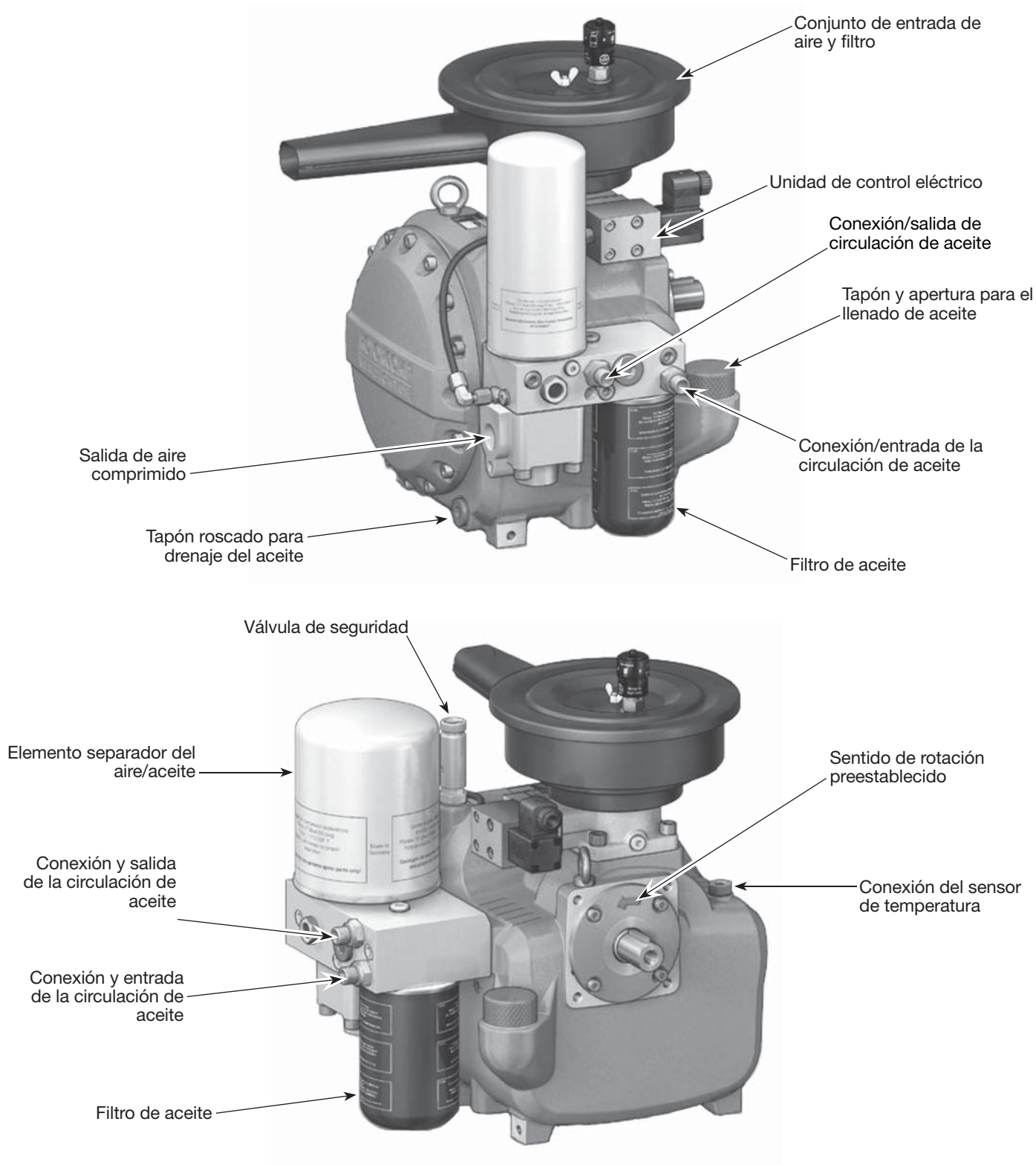
Figura 3 - Componentes de la unidad de compresión
