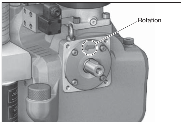
Figure 6 - Sens de rotation
