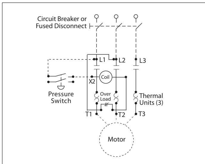
Figure 7 - Diagrama de cableado trifásico
