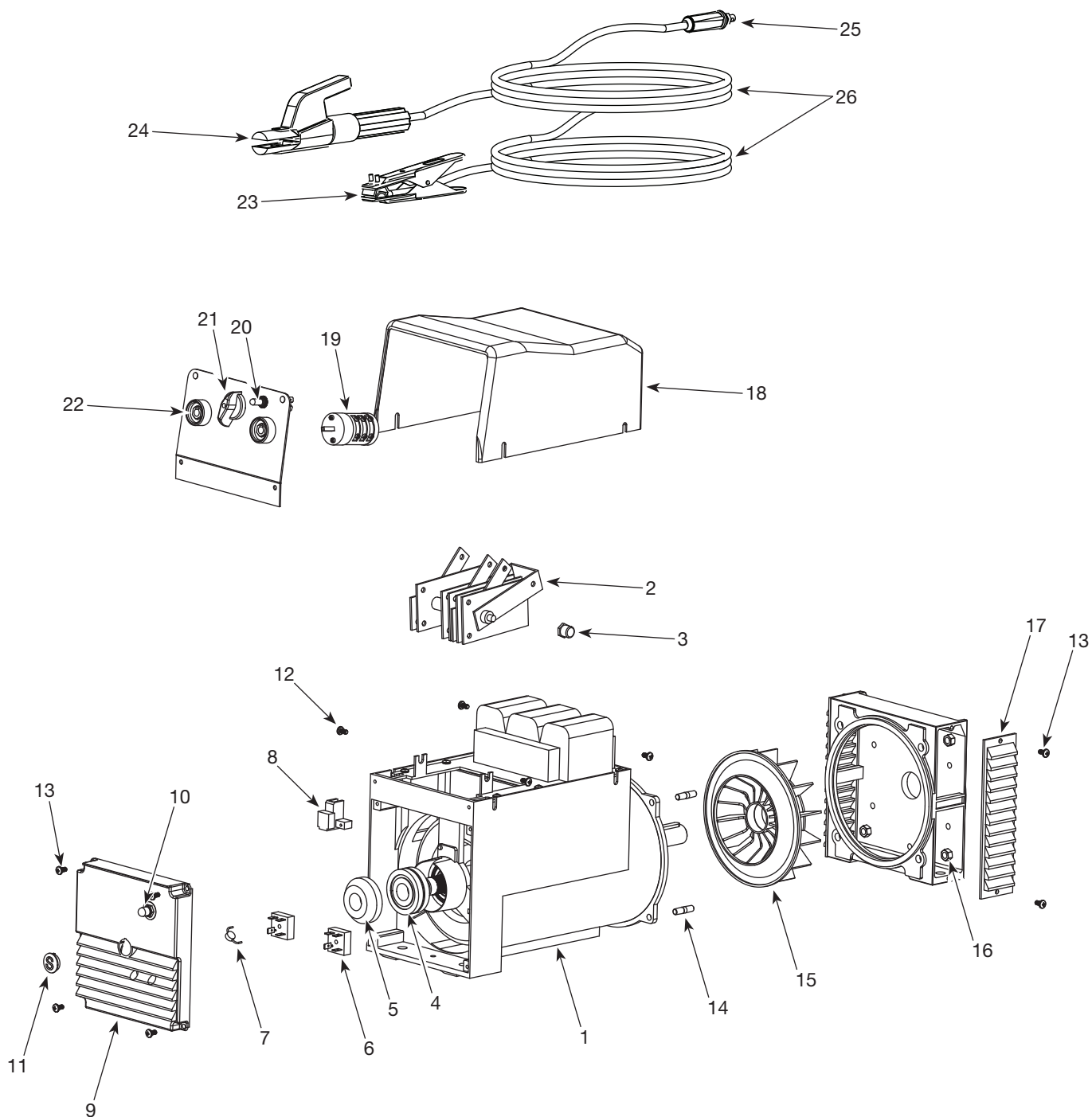
Figura 16 - Conjunto del alternador (GW004996AV se muestra)
