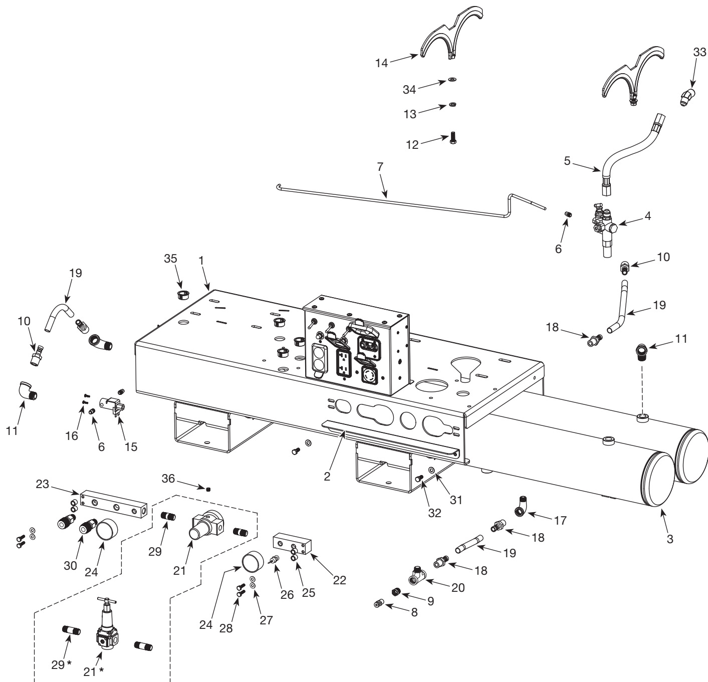
Figura 13 - Se muestra el conjunto del chasis para el GR2100 y el GR3100; las piezas en común para todos los modelos se muestran en la lista de partes de la Figura 13.
