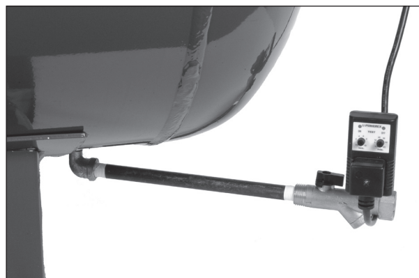
Figure 17 - Drenaje automático del tanque
