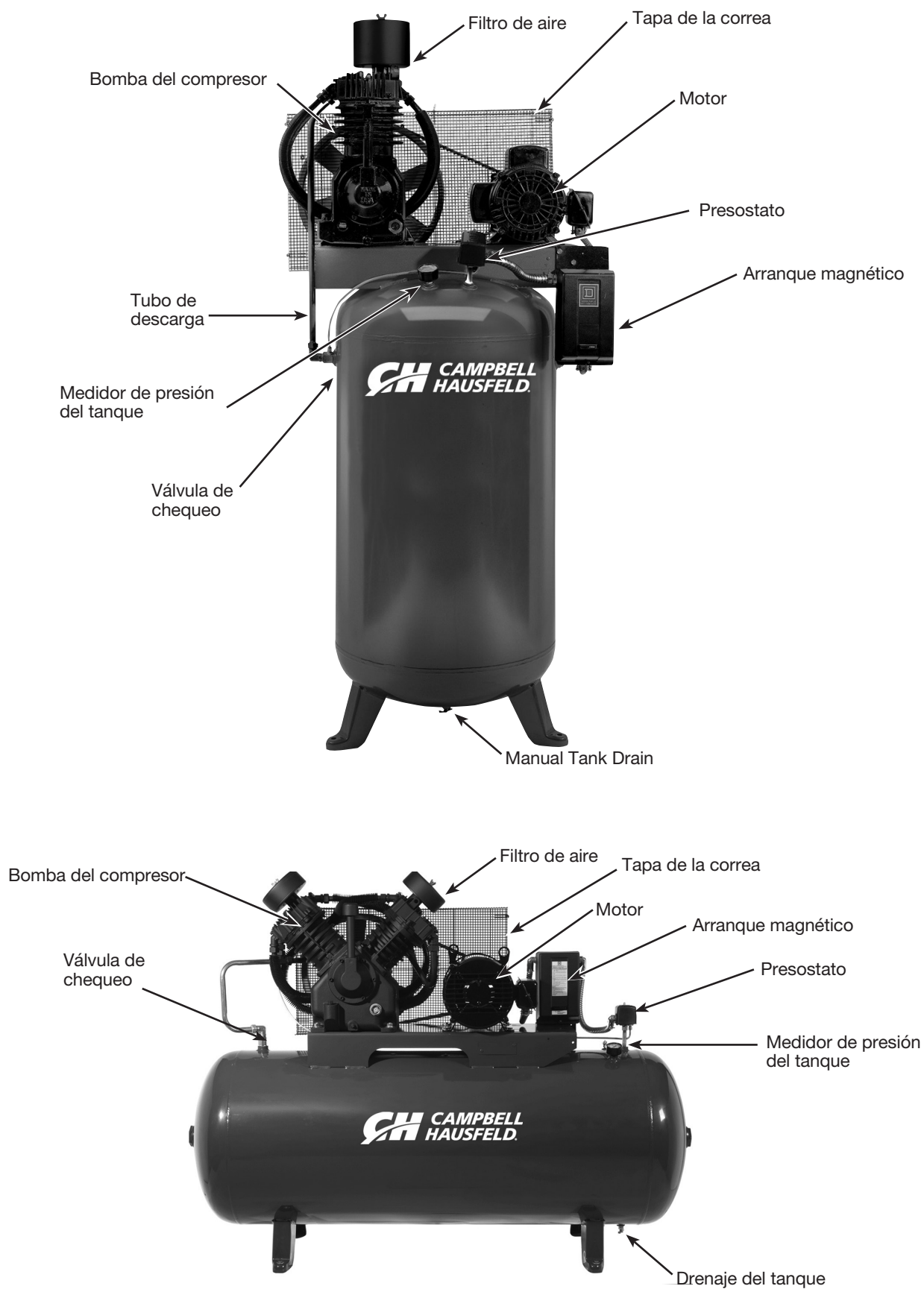
Figura 1 - Componentes de la serie de taller
