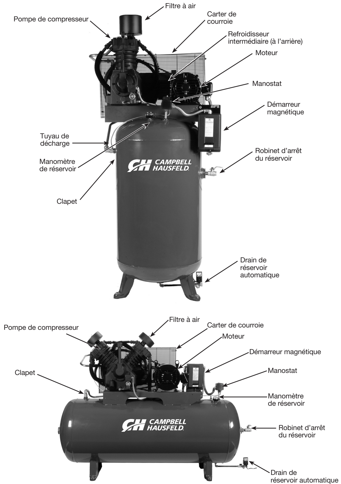
Figure 2 - Composants de la série Pneu et lubrifiant
