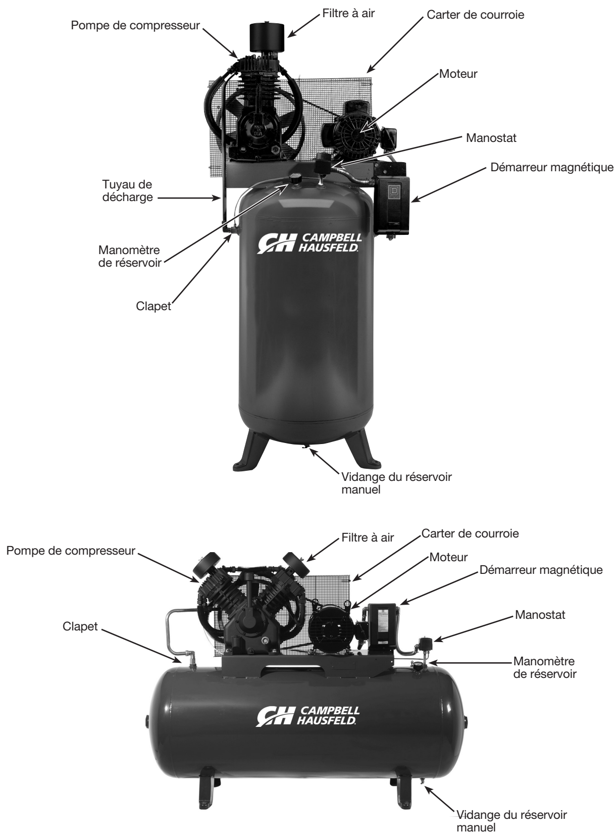
Figure 1 - Composants de la série Air d'atelier
