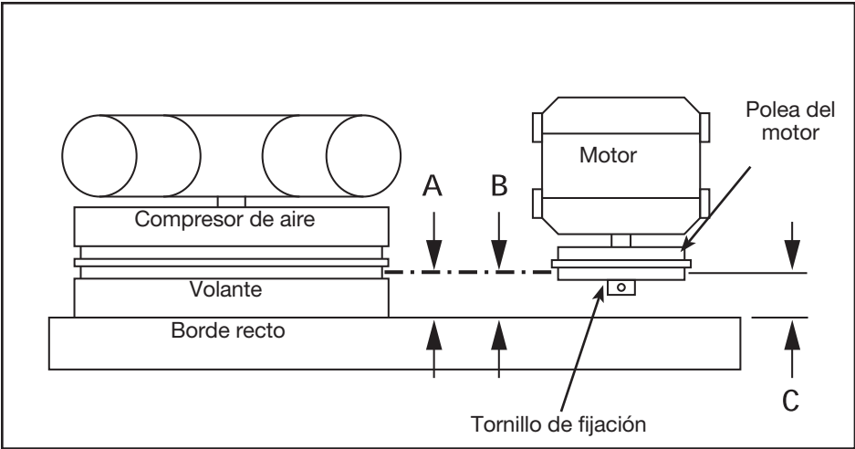
Figura 20 - Vista superior
