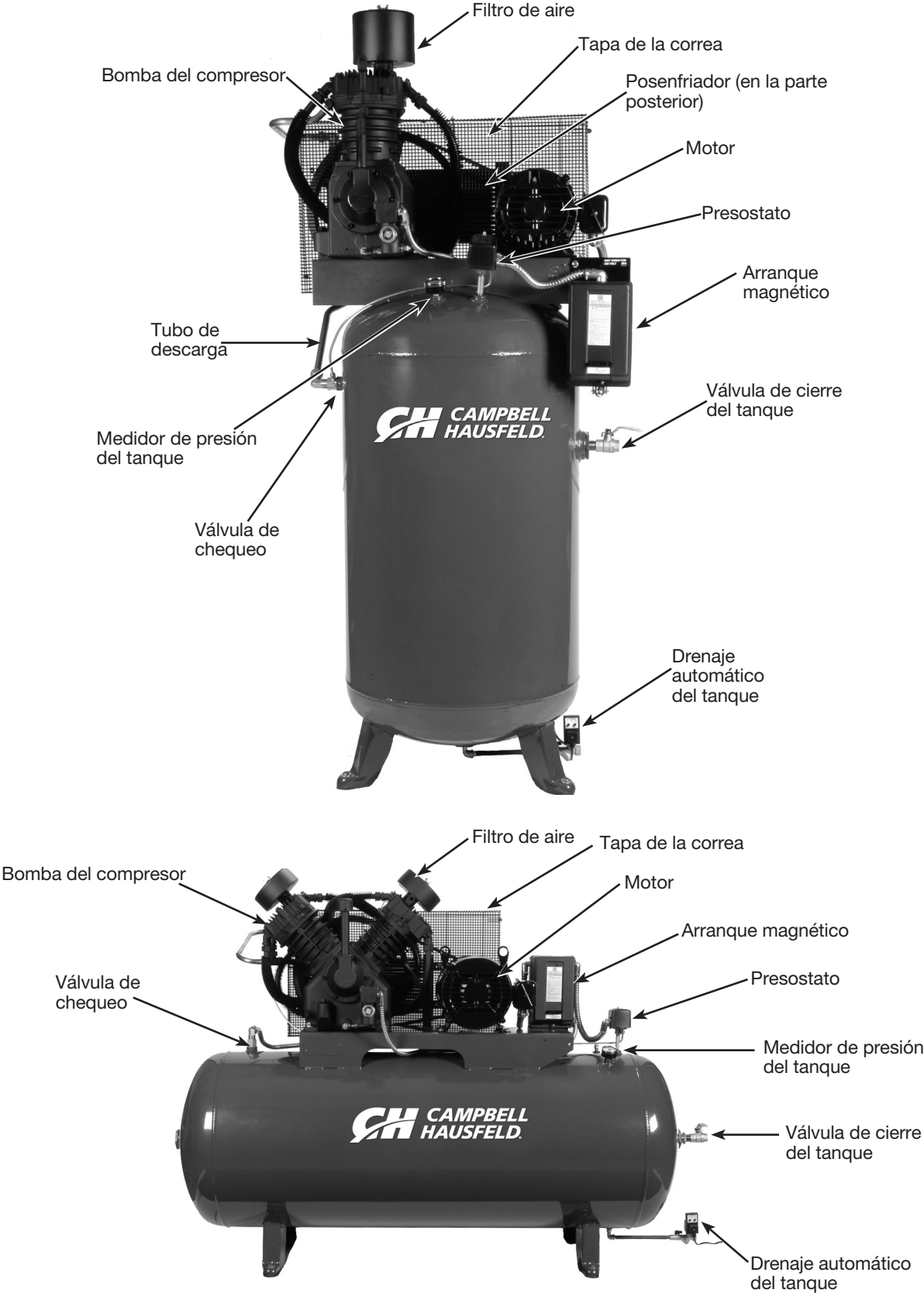
Figura 2 - Componentes de la serie de neumáticos y lubricantes
