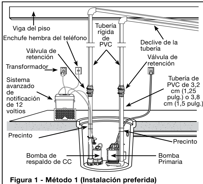
Figura 1 - Método 1 (Instalación preferida)
