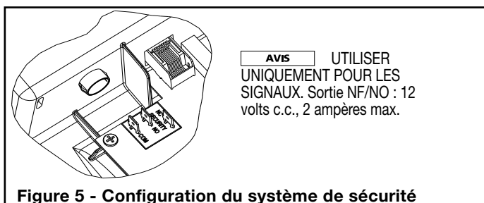
Figure 5 - Configuration du système de sécurité
