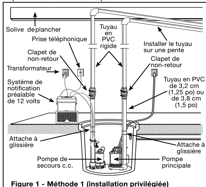
Figure 1 - Méthode 1 (installation privilégiée)
