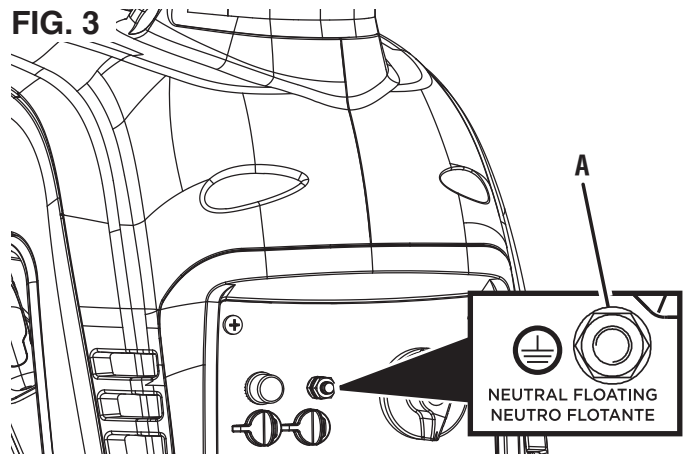
A - Terminale à la terre
