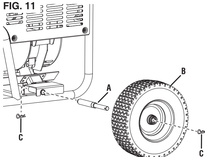
A - Essieu B - Roue C - Goupille d'attelage
