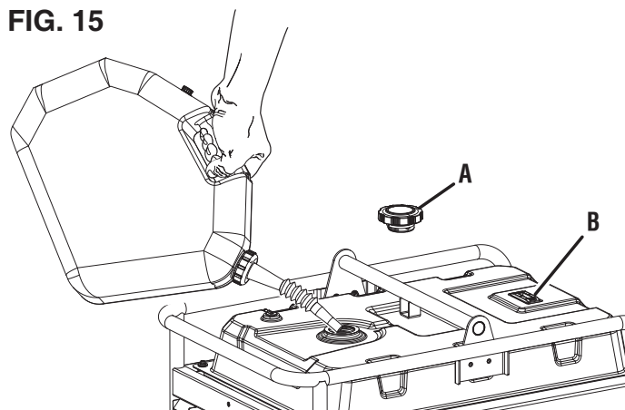
A - Bouchon de réservoir B - Jauge de carburant
