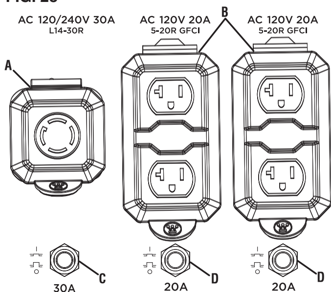
A - 120/240 volt AC 30 amp receptacle
