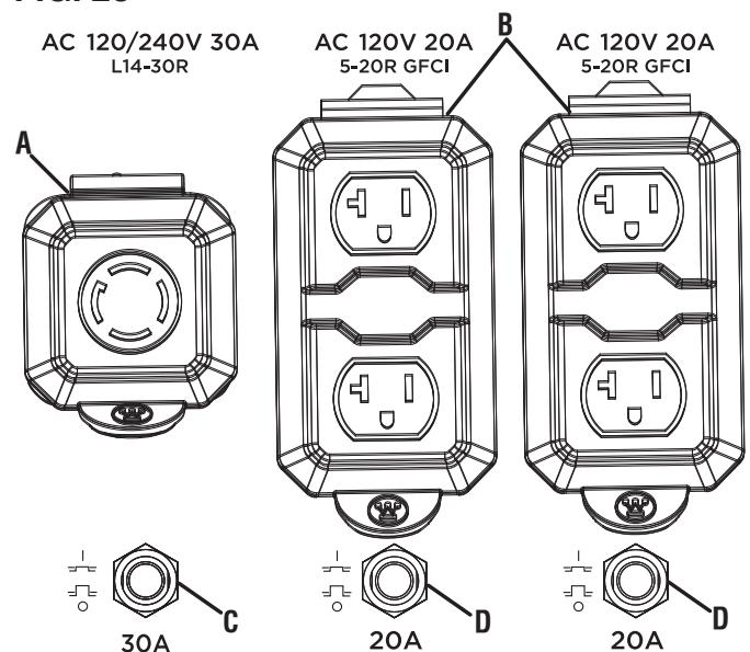
A - Prise 120/240 volts CA 30 ampères
