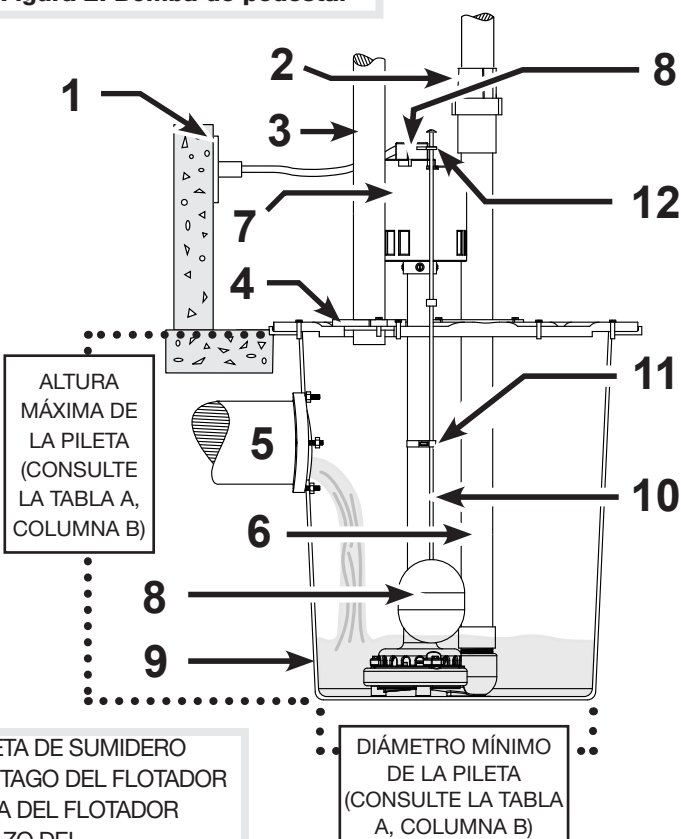
Figura 2: Bomba de pedestal
