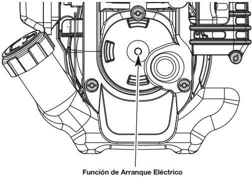
Función de Arranque Eléctrico
