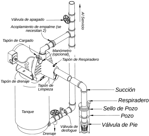
Fig.2d POZO POCO PROFUNDO - SISTEMA MONTADO EN EL TANQUE (CON VÁLVULA DE PIE)
