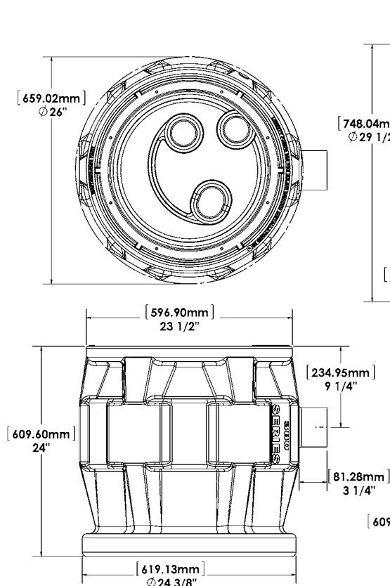
Données sur les dimensions : Modèles PRO380 simples
