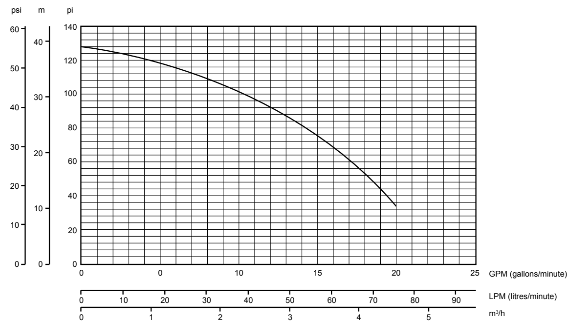
Annexe 1 : Courbe de rendement du système de surpression Inline
