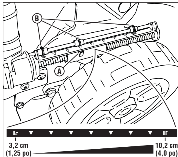
Figure 7 : Indicateur de hauteur de coupe
