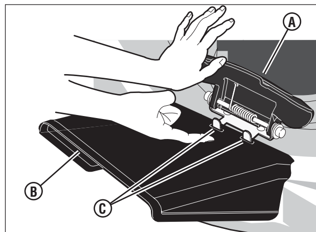
Figure 8 : Installation du déflecteur d'éjection
