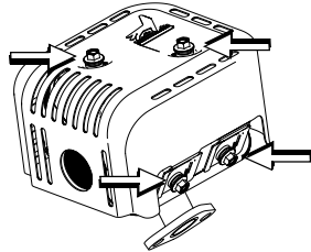
Figura 3-20. Sujetadores del blindaje contra calor
