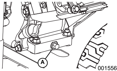
Figura 4-7. Tapón de vaciado de aceite
